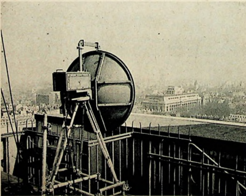
BEGINPUNT VAN DE LINK (links onder) - Hier ziet men de op het dak van het Senate House te Londen opgestelde zender, die de beeldsignalen doorgaf naar Wrotham.
